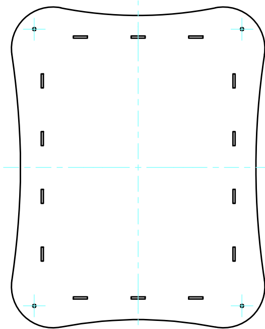
下カバー表面 / Bottom cover Frontside
